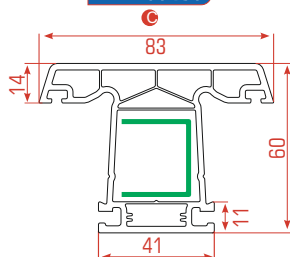
Poste T
