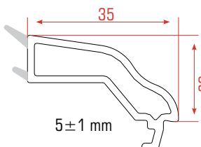
Monolitico Junquillos
