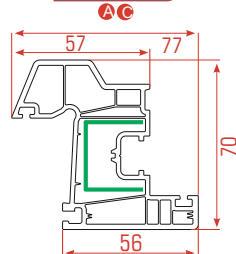
Drainaged Hoja Fijo
