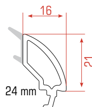
Doble Junquillos
