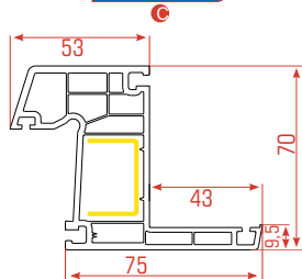
Renovación Marco fijo
