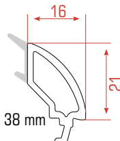
Junquillos
