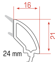
Doble Junquillos
