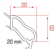
Doble Junquillos
