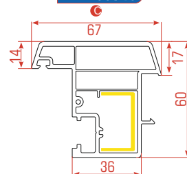
Poste Batiente
