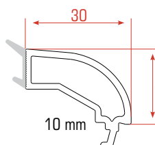
Monolitico Junquillos
