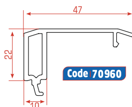
Tapa Junquillo
