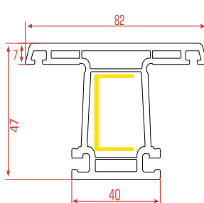
Poste T corredera
