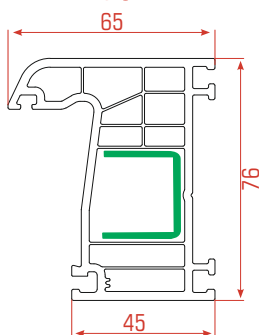
Marco Fijo
