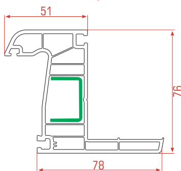
Renovación Marco fijo
