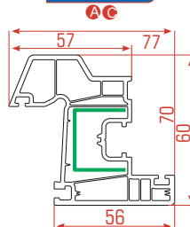
Drainaged Hoja Fijo
