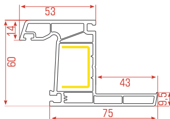
Renovación Marco fijo
