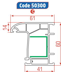
Marco Fijo
