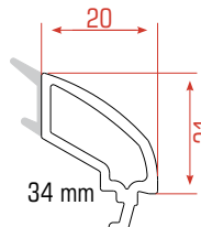
Junquillos
