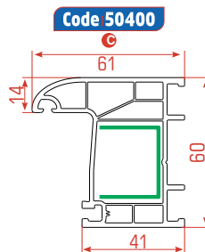
Marco Fijo
