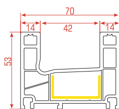
Marco Corredera Doble Riel
