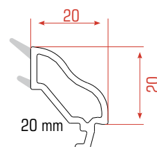
Doble Junquillos
