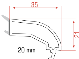
Junquillos
