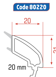
Doble Vidrio Junquillos
