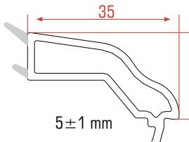
Monolitico Junquillos
