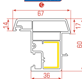
Perfil Traslapo Falso
