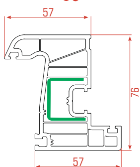
Hoja Fijo
