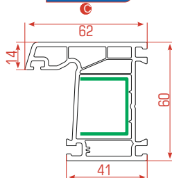
Narrow Marco Fijo
