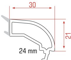
Junquillos
