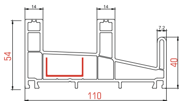
Marco Doble Riel Corredera Para Moscas
