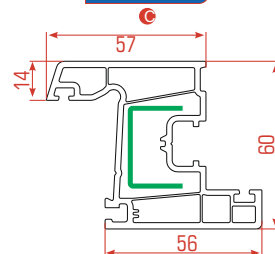
Hoja interior
