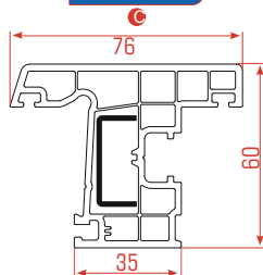
Hoja Ventana Exterior
