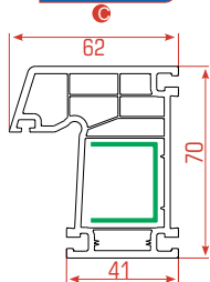
Marco Fijo
