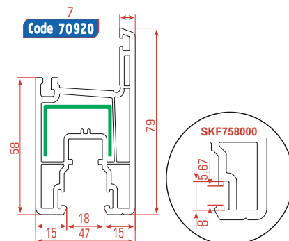
Hoja Corredera
