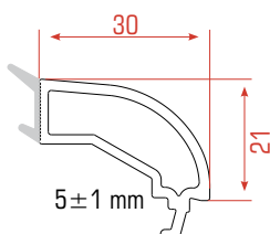
Solo Junquillos
