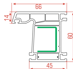
Marco Fijo
