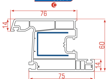
Hoja Puerta Interior
