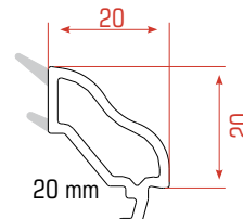
Doble Junquillos
