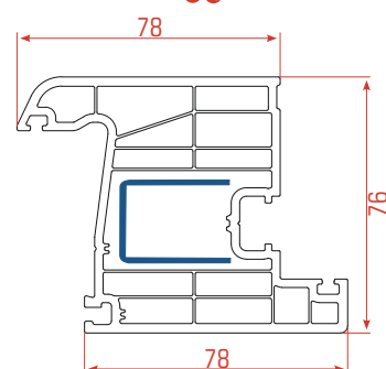
Hoja Puerta Interior
