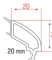
Doble Junquillos
