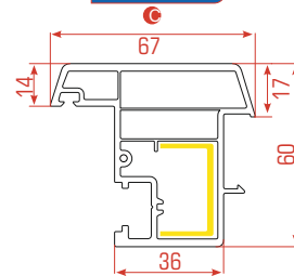
Perfil Traslapo Falso
