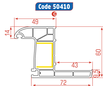
Renovación Marco fijo
