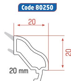
Doble Vidrio Junquillos
