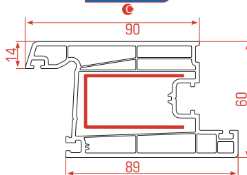
Hoja Puerta Interior Grande
