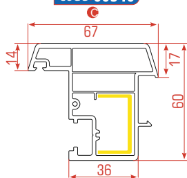
Perfil Batiente
