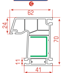
Marco Fijo
