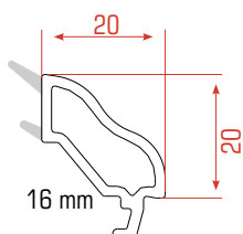
Doble Junquillos
