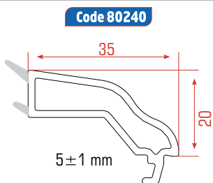
Solo Vidrio Junquillos
