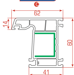
Marco Fijo
