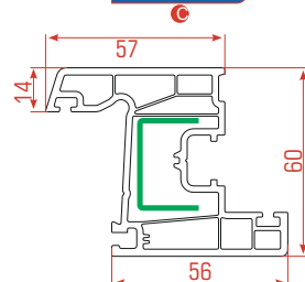
Hoja Fijo
