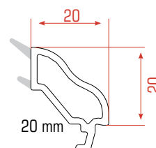
Doble Junquillos
