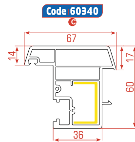
Perfil Traslapo Falso
