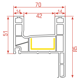
Renovation Sliding Marco Fijo
