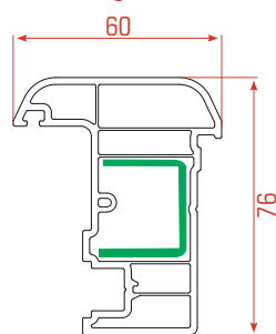
Perfil Traslazo Falso
