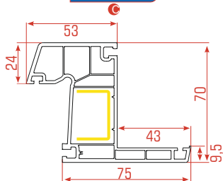
Renovación Marco fijo
