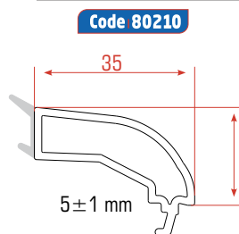
Monolitico Junquillos
