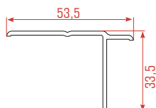
Perfil de T PVC
