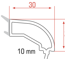
Monolitico Junquillos
