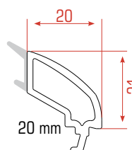
Doble Junquillos
