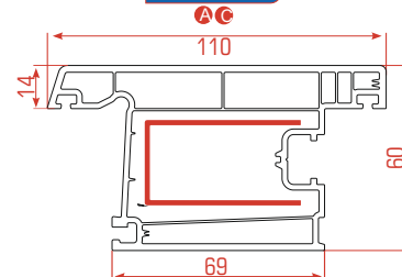
Hoja Puerta Exterior
