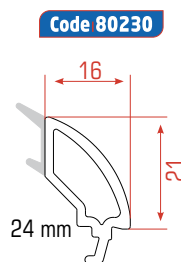
Doble Vidrio Junquillos
