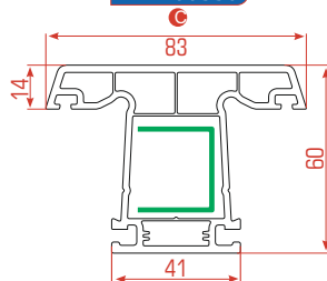
Poste T
