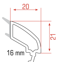
Doble Junquillos
