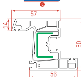
Hoja Interior
