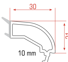
Monolitico Junquillos
