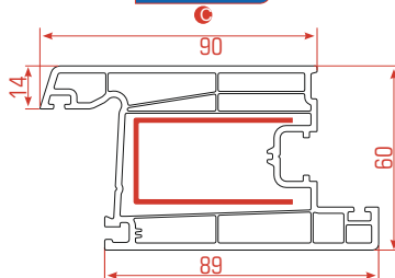
Hoja Puerta Interior
