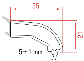
Monolitico Junquillos
